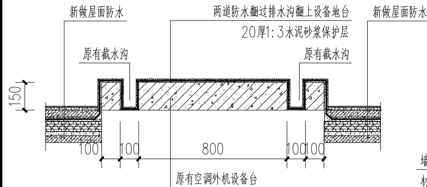
④ 空调外机设备地台防水处理大样 1:20
