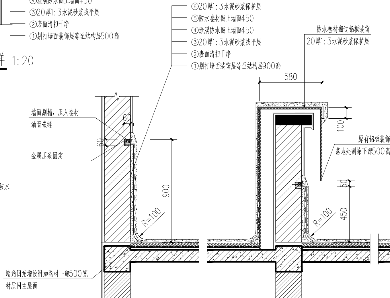
② 不上人屋面防水大样 1:20
