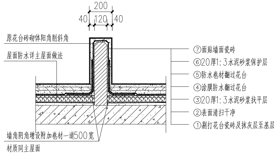
③ 保留原有花台防水处理大样 1:20
