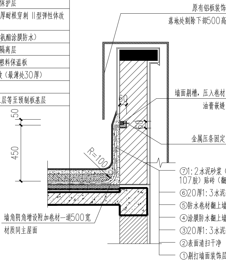
① 上人屋面防水A、B大样 1:20
