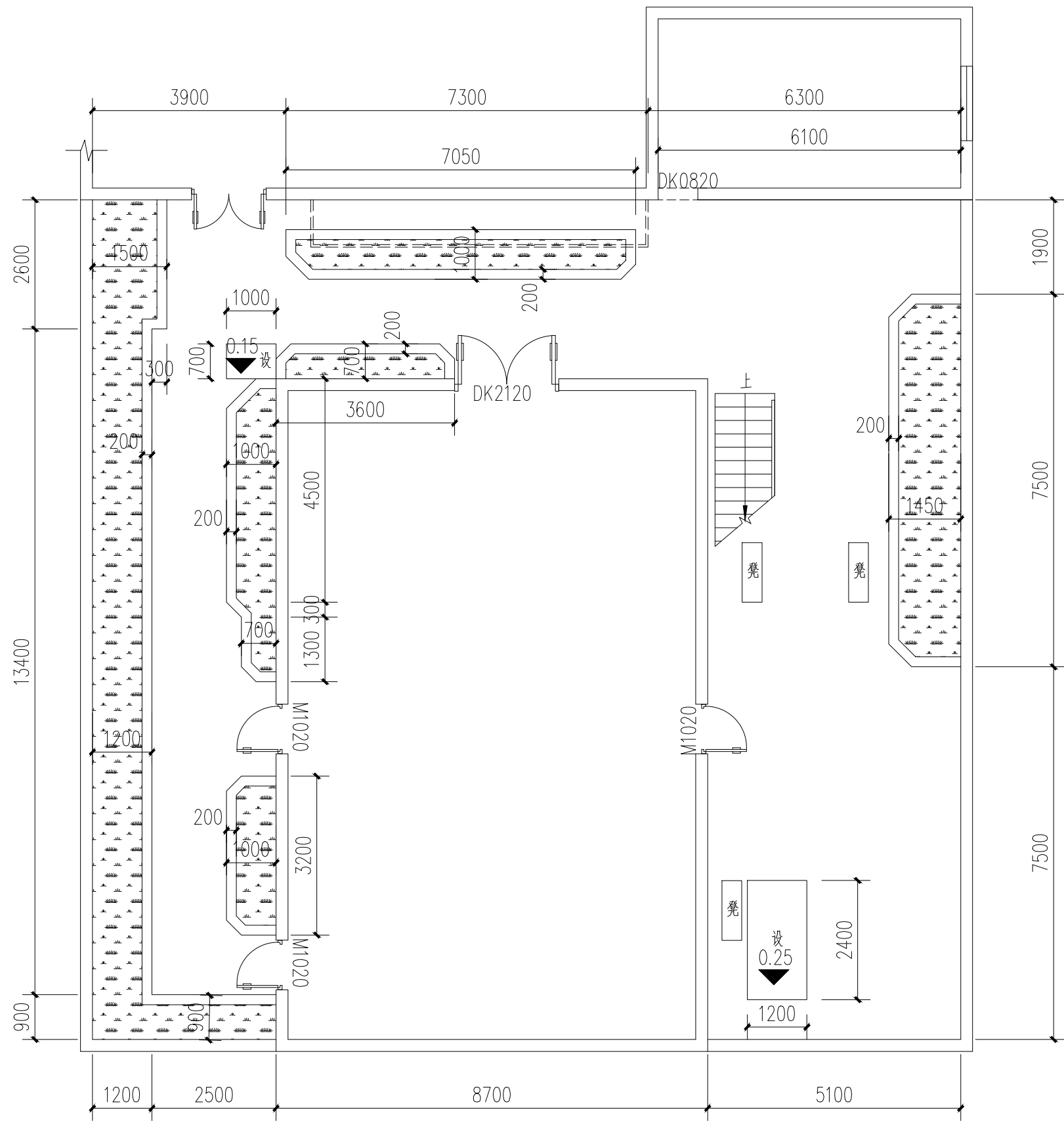
屋面一层尺寸平面图 1:100
