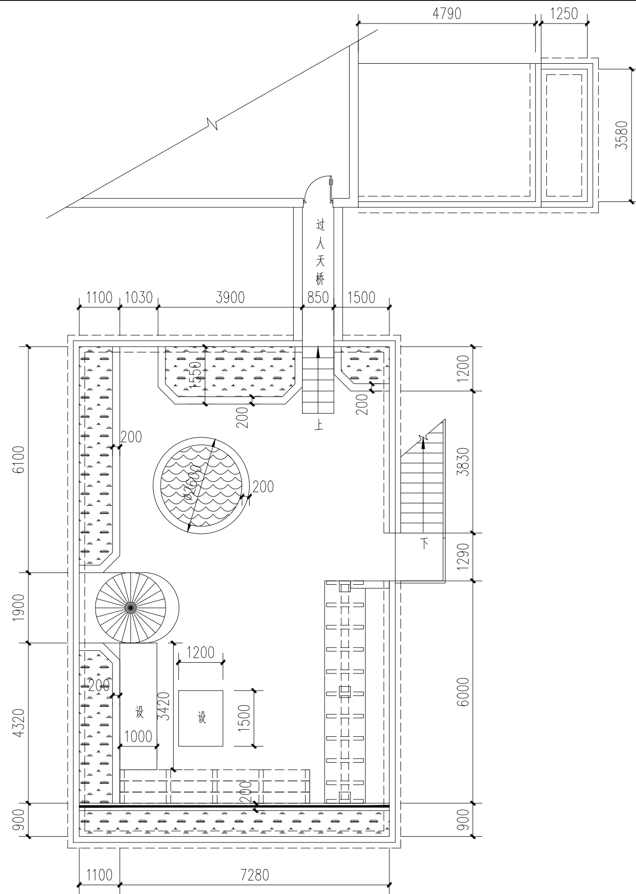
屋面二层尺寸平面图 1:100
