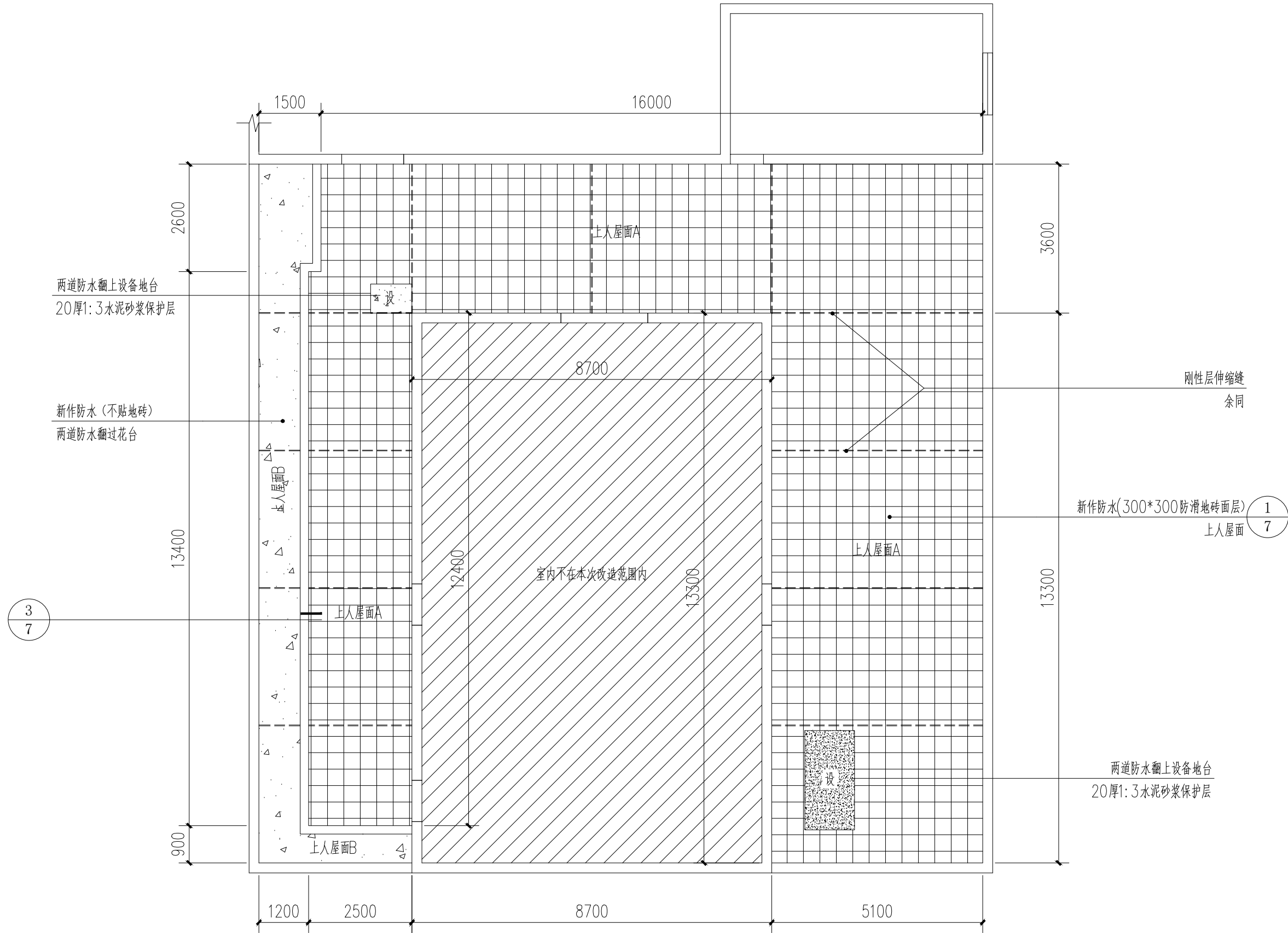
屋面一层防水平面图 1:100
