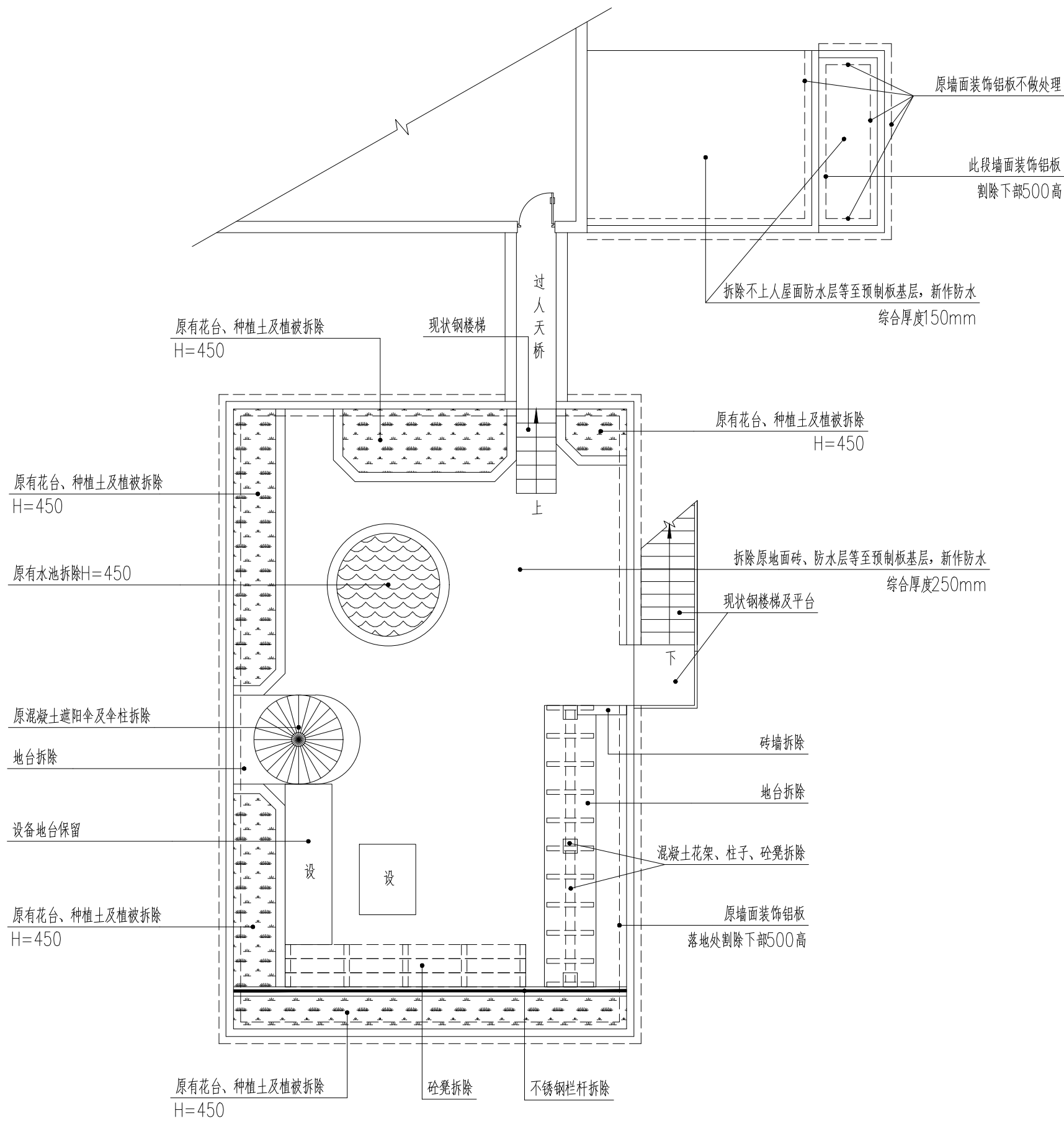
屋面二层改造平面图 1:100
