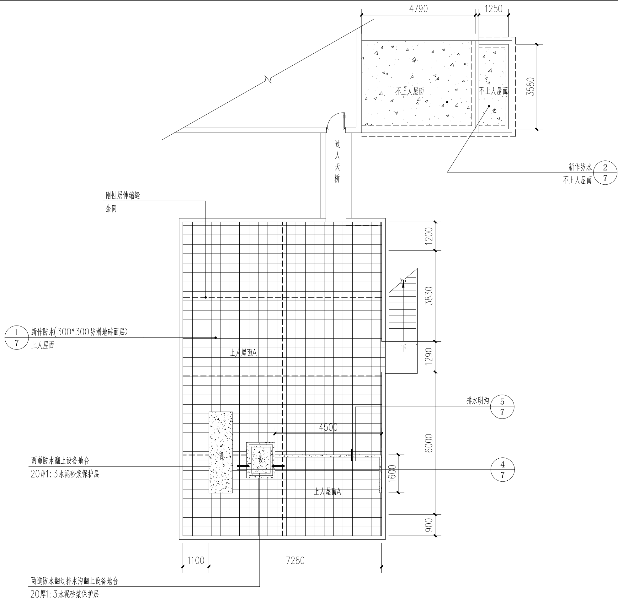
屋面二层防水平面图 1:100
